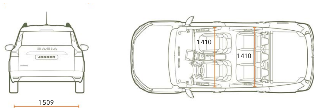
5-KOHALINE VERSIOON
