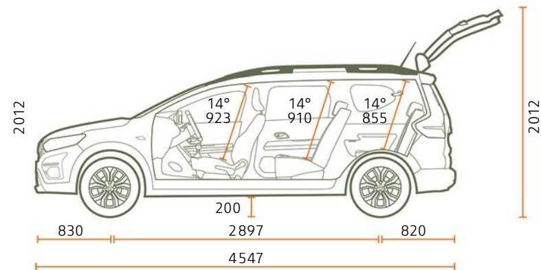
7-KOHALINE VERSIOON
