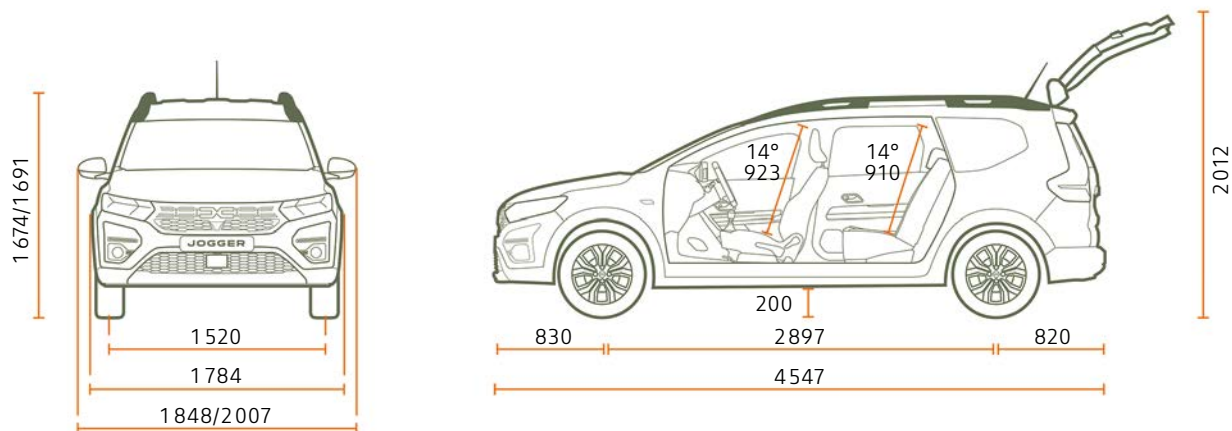
5-KOHALINE VERSIOON
